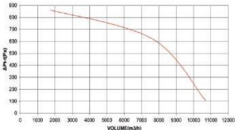
Φ350-4.0HP-1450RPM
