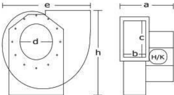
Φ350-4.0HP-1450RPM
